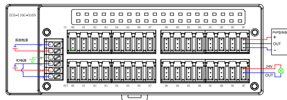
EC6-I16C-O16N (PNP输入, NPN输出)
