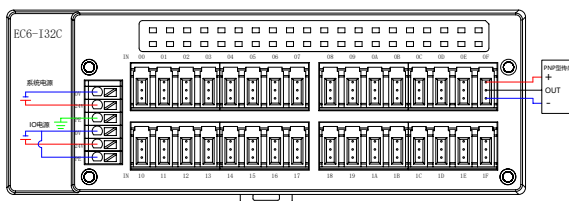
EC6-I32C (PNP输入)
