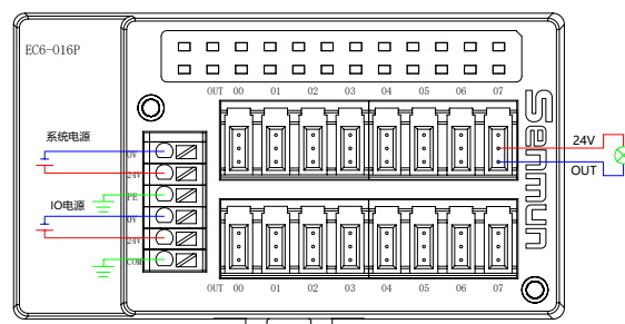
EC6-O16P (PNP输出)
