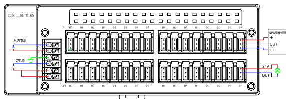
EC6-I16C-O16N (NPN输入, NPN输出)
