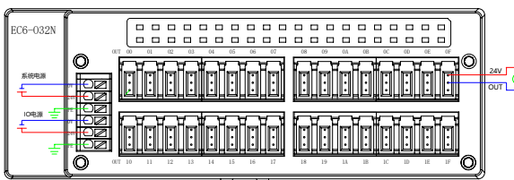
EC6-O32N (NPN输出)
