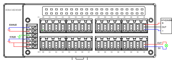
EC6-I16C-O16P (NPN输入, PNP输出)
