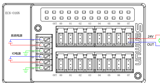
EC6-O16N (NPN输出)
