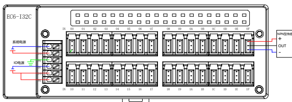
EC6-I32C (NPN输入)
