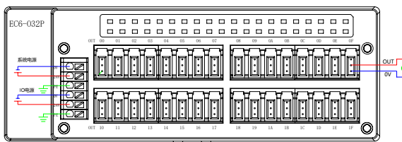
EC6-O32P (PNP输出)
